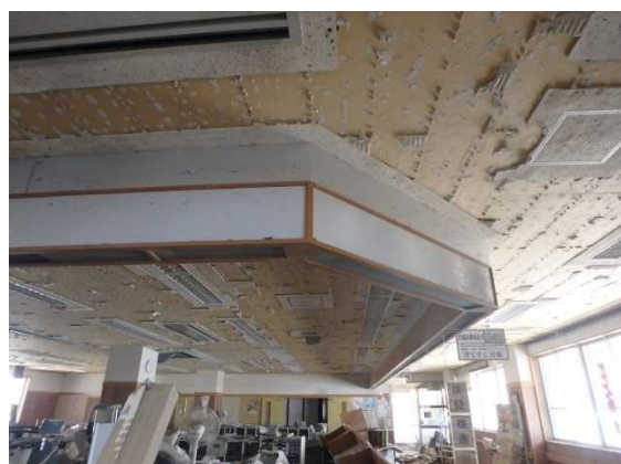
水没後に落下したロックウール吸音天井板
