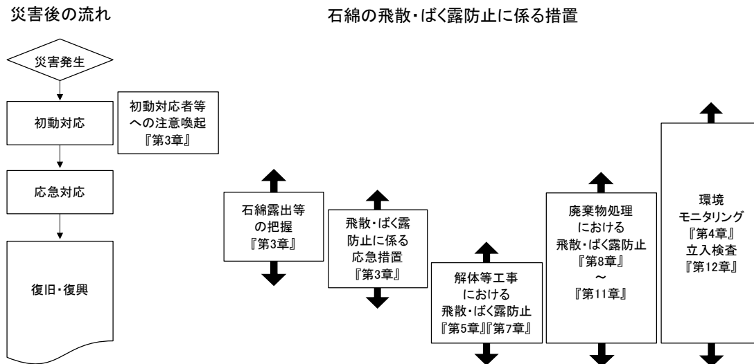
図 2.7 石綿の飛散・ばく露防止に係る実施事項のタイムテーブル(例)
